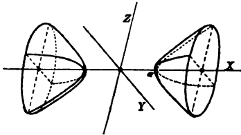
C. 1877. Hyperboloid dvojitý.
